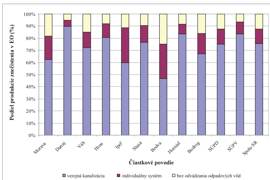
Obr. 4.2 Spôsoby odvádzania komunálnych odpadových vôd z aglomerácií nad 2 000 EO – rok 2005
