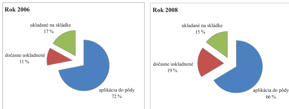
Obr. 4.3 Nakladanie s kalom z ČOV vodárenských spoločností SR v rokoch 2006 a 2008
