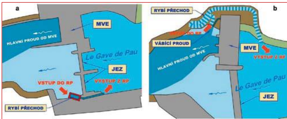
Obr. 166 a (vľavo) – príklad nevhodného umiestnenia rybovodu, Obr. 166 b (vpravo) – príklad vhodného umiestnenia rybovodu (Larinier 2005, upravené podľa Slávik et al. 2012).
