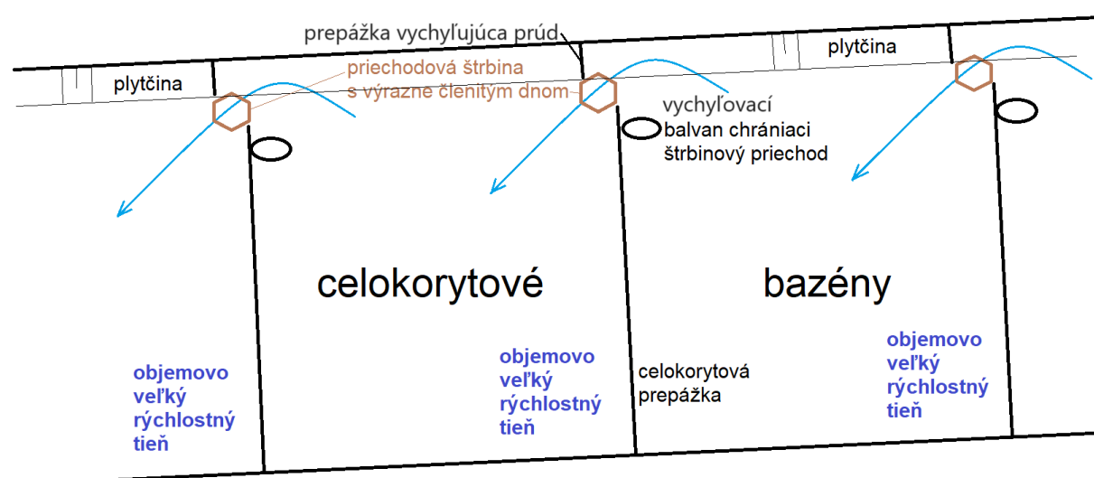
Obr. 24 Príklad riešenia celokorytových bazénov, ústretového pre drobné ryby a bentos.
