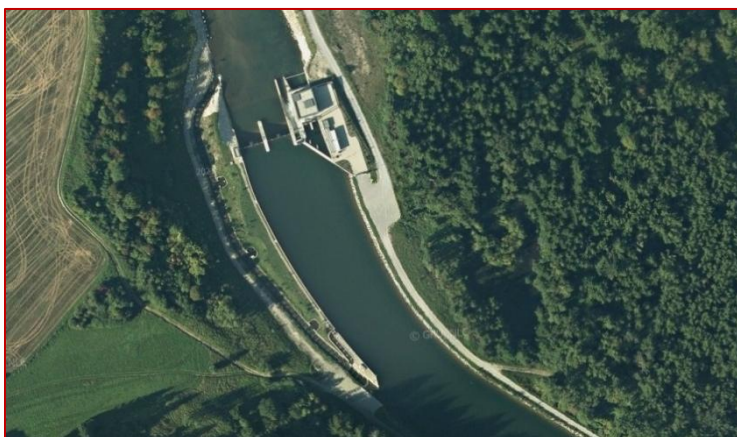
Obr. 125 Poloha obtokového bazénového rybovodu pri zdrži MVE Podtureň - Liptovský Ján. (zdroj ZBGIS)
