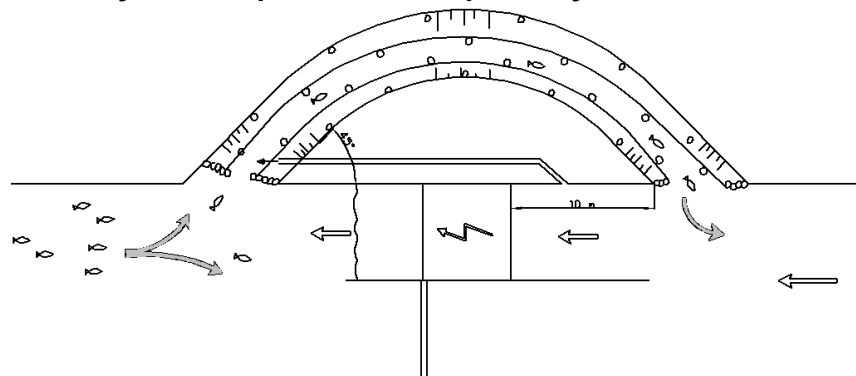
Obr. 190 Schéma obtokového bystrinného spriechodnenia.
