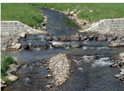
Typ 5: Celokorytové bazény.
