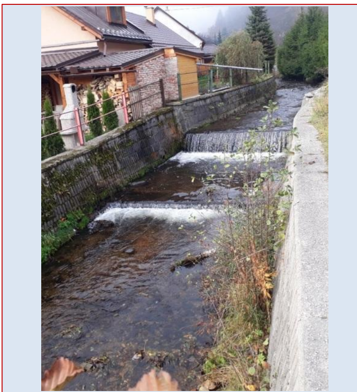
Obr. 72 Pôvodná nepriechodná migračná bariéra pred spriechnením - vodopádové stupne v dne.
