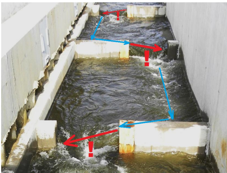
Obr. 107 Pohľad na komory pred osadením balvanov – vždy jedna rýchla prúdnicca popri brehu narážala na stenu prepážky a zboku vrážala do priechodového otvoru (vážna hydraulická komplikácia pre ryby, namáhavo prekonávajúce prechod skokovou alebo maximálnou rýchlosťou).
