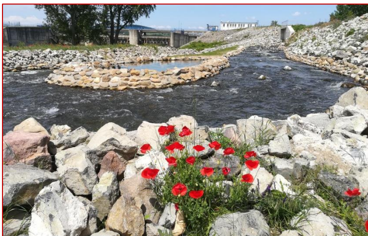
Obr. 93 Pohľad na dolný úsek bystriny medzi Hronom a protipovodňovou hrádzou, s 1. oddychovou zátokou. Tento úsek je skrátený kvôli vyústeniu kanalizácie, a teda strmší (1:50), má však po celej trase spomalené okrajové plytčiny. Je prelievaný povodňami, preto je podbetónovaný.
