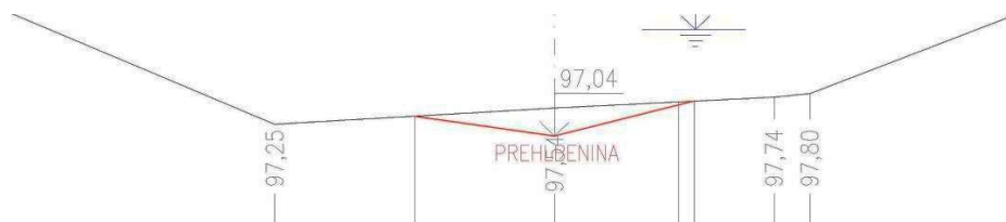
Obr. 53 Priečný rez prehĺbeniny (náhradnej hĺbočiny) pod sklzom.
