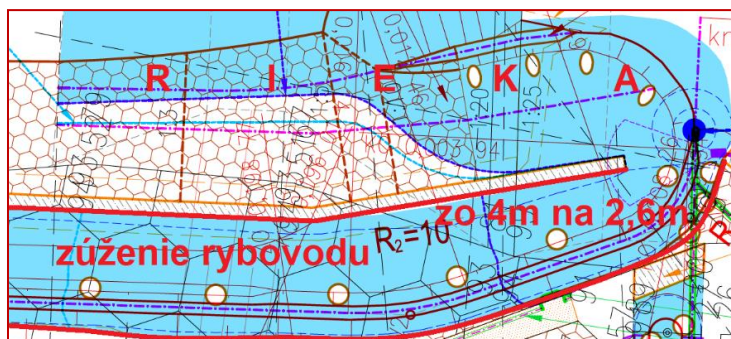
Obr. 22 vľavo (schéma vyústenia rybovodu hať Martin tok Turiec) a Obr. 23 vpravo (VD Petershagen tok Weser) Príklady potrebnej koncentrácie vábiaceho prúdu priamo na výtoku z rybovodu do hlavného toku, ktorým migrujú ryby: vľavo zúženie výtoku z rybovodu zo 4 m na 2,6 m, vpravo obrázok z metodiky Slavík a kol. 2012, kde však potrebné zúženie odporúčame vyriešiť prírode bližším spôsobom – napr. prerušeným radom balvanov alebo zúžením brehov rybovodu v ústí do rieky.
