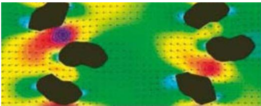
Obr. 132 Príklad rozloženia rýchlostí vody pri pretekaní mnohomedzerovou líniou balvanov - 2D matematický model prúdenia vody. Hlavný prúd tečie sprava doľava, svetlomodré sú tíšiny, bodové maximum rýchlosti vody je červené až fialové. Tieto mnohomedzerové priečne línie balvanov, ktoré len trochu zavzdúvajú a pribrzdžujú prúd vody v rybovode, pričom za každým balvanom vzniká len veľmi malý priestor rýchlostného tieňa, teda nevytvárajú rozsiahlejšie pokojnejšie miesta v rybovode. (Slavík a kol. 2012).
