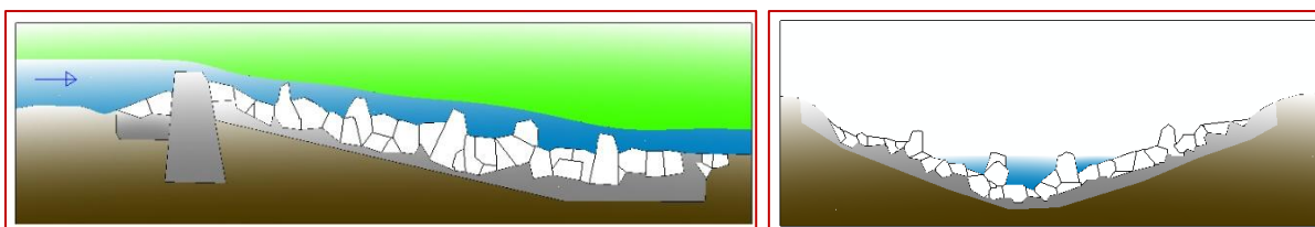
Obr. 181 Sklz so zníženým pôvodným prahom a celoplošne spevneným podkladom.
