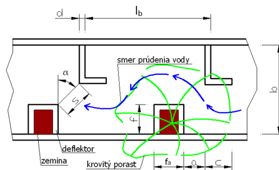
Obr. 198 Pôdorysná schéma štrbinového rybovodu.
