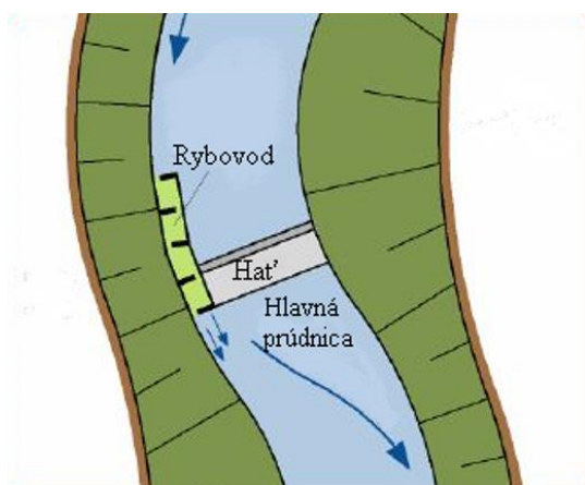
Obr. 13 vľavo (Larinier 1992b) Obr. 14 vpravo (DWA-M 509 foto: Dumont) Príklady správneho umiestnenia vstupu do rybovodu v úrovni migračnej bariéry, nie poniže nej, tiež pri nárazovom brehu, nie pri usadzovacom.
