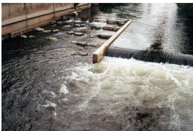
Obr. 13 vľavo (Larinier 1992b) Obr. 14 vpravo (DWA-M 509 foto: Dumont) Príklady správneho umiestnenia vstupu do rybovodu v úrovni migračnej bariéry, nie poniže nej, tiež pri nárazovom brehu, nie pri usadzovacom.
