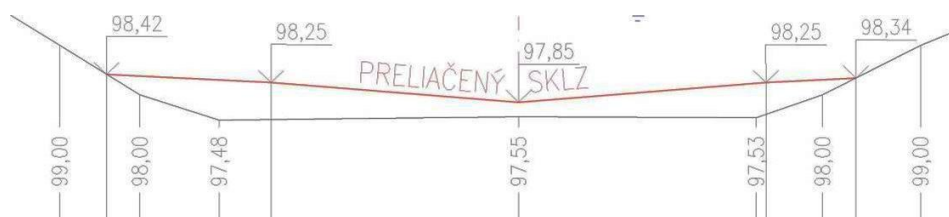
Obr. 52 Priečný rez v strede trasy, kde bolo nutné výrazne dosypať terén nad pôvodným dnom.
