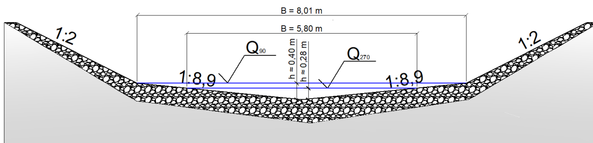
Obr. 185 Schéma návrhu úpravy profilu priepadu kamenného sklzu návrh I.
