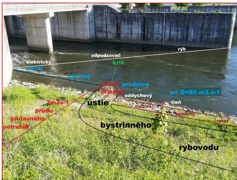
Obr. 87 Návrh optimálneho ústia preložky rybovodu Žilina do vodiaceho prúdu Váhu pod turbínami, podľa výsledkov ichthyomonitoringu 2020.
