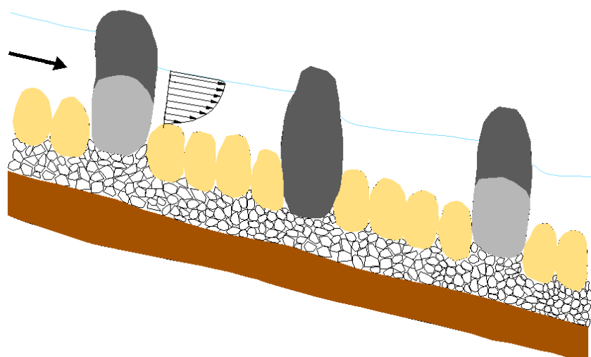
Obr. 25 a Schematické znázornenie výrazne znížených rýchlostí pri členitom dne rybovodu. Preto proti výrazne pomalšiemu prúdu popri členitom dne môžu preplávať aj menej zdatné malé ryby, hoci proti maximálnej „povolenej“ rýchlosti vody popri hladine by to nedokázali.
