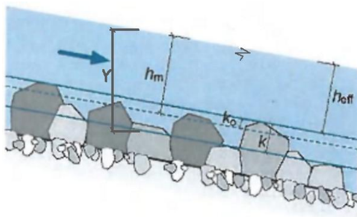
Obr. 177 Schéma určenia hĺbky toku h_m (DWA M-905).
