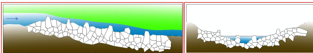
Obr. 180 Sklz s odstráneným prahom celoplošne nespevnený .
