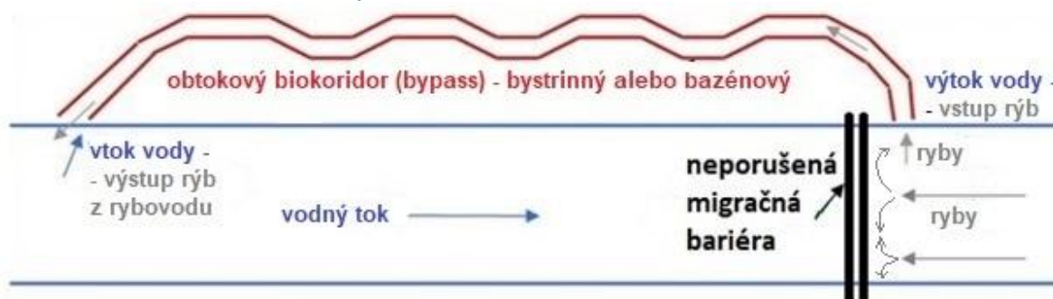
Obr. 4 Pôdorys obtokového biokoridoru (bypassu) – bystrinného alebo bazénového.
