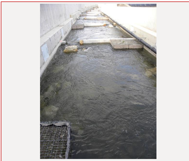
Obr.104 Pohľad na druhú a tretiu štvrtinu rybovodu, širokú až 6 m, už s vlastnosťami „oddychových“ bazénov.
