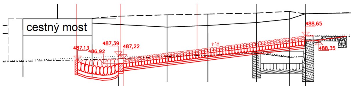
Obr. 74 Pozdĺžny rez pôvodným stupňom (mierne odstráneným do trojuholníkového profilu), celokorytovým sklzom a náhradnou hĺbočinou pod ním (už pod cestným mostom).
