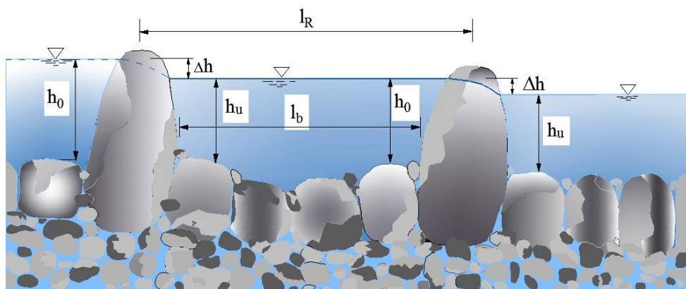
Obr. 205 Geometria bazéna v pozdĺžnom reze (Fischauftstiegsanlagen in Bayern, 2012).
