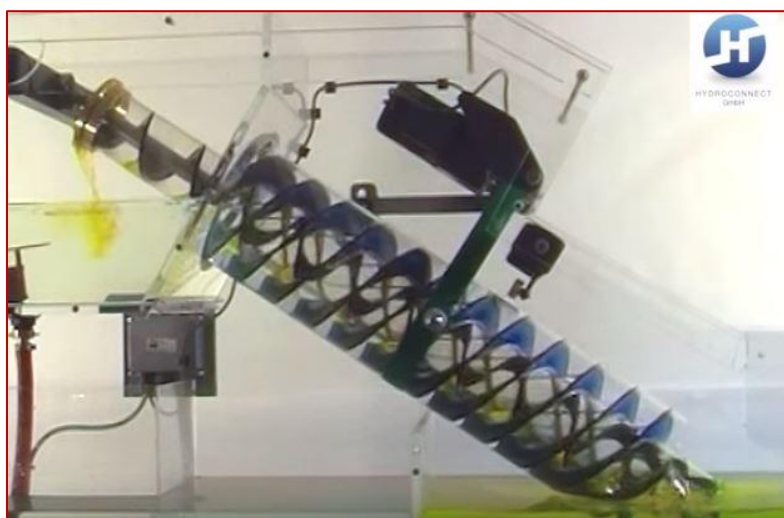
Obr. 164 Model dlhšieho vnútorného potrubia, vytlačajúceho vodu s rybami z dolnej hladiny do hornej, počas farbacej skúšky (žltá voda), a kratšieho vonkajšieho potrubia, zabezpečujúceho pohon a poprúdovú migráciu. (Hydro-Connect GmbH)
