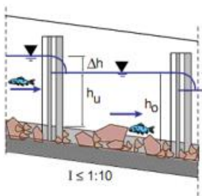
Obr. 199 Pozdĺžny rez bazénom štrbinového rybovodu. Obr. 200 Grafická závislosť \mu_v od podielu h_u/h_o .
