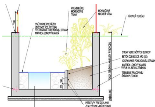
Obr. 33 a vľavo Príklad vegetačných zemných boxov v projekte (rybovod Zvolen) a Obr. 33 b vpravo Realizované zazemnené boxy v bazénovom rybovode Šalková po 6 rokoch prevádzky.
